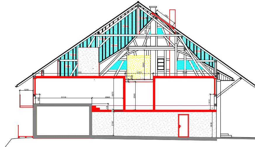
Schnitt 2
