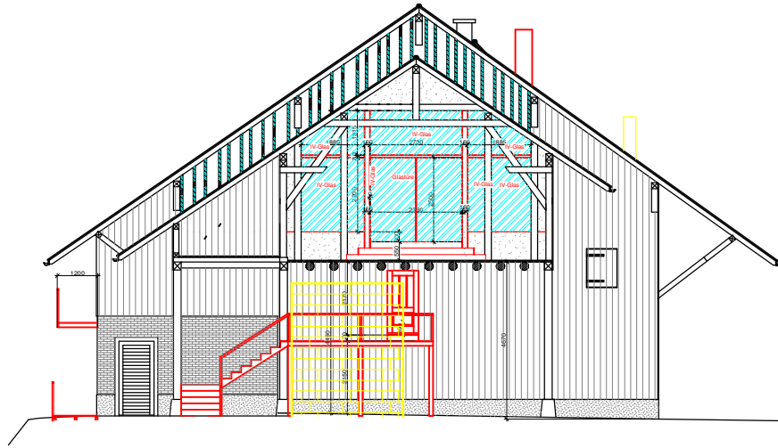
Schnitt 1
