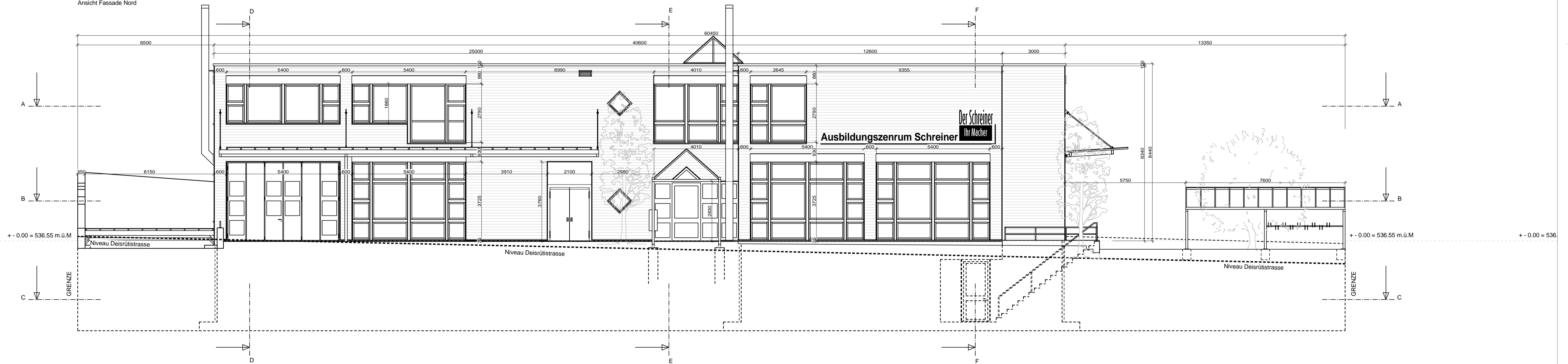
Ansicht Fassade Nord
